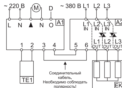
Схема подключения вентилятора и нагревателя на 400 В/ 3 фазы мощностью до 16(26)-ти кВт к терморегулятору MPT.380.16-25(40)*
