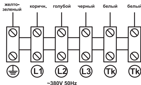
Схема подключения №4
