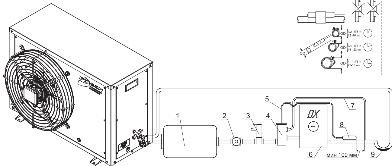
Схема установки термобаллона ТРВ
