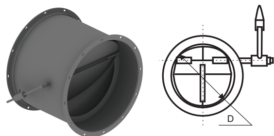
Клапаны из углеродистой стали
