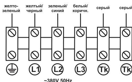
Схема подключения №7
