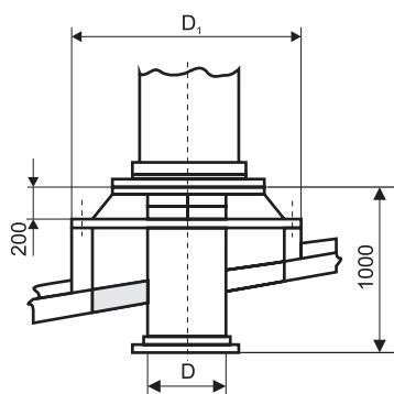
Узел прохода без клапана УП1
