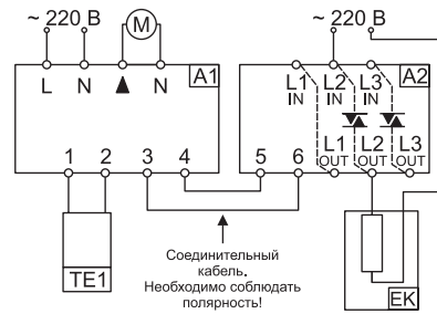
Схема подключения вентилятора и нагревателя на 220 В мощностью до 5(8)-ти кВт к терморегулятору MPT.380.14-25(40) к сети 220 В*
